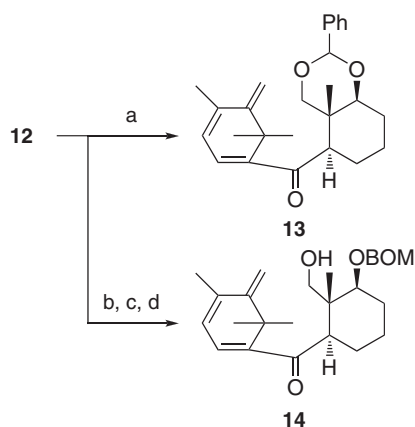
Scheme 3. Preparation of ketones 13 and 14 . (a) PhCH(OMe) 2 , CSA, CH 2 Cl 2 , 52%; (b) TBSCl, imidazole, CH 2 Cl 2 ; (c) BOMCl, i -Pr 2 NEt, CH 2 Cl 2 ; (d) TBAF, THF, 3 steps 47%.
